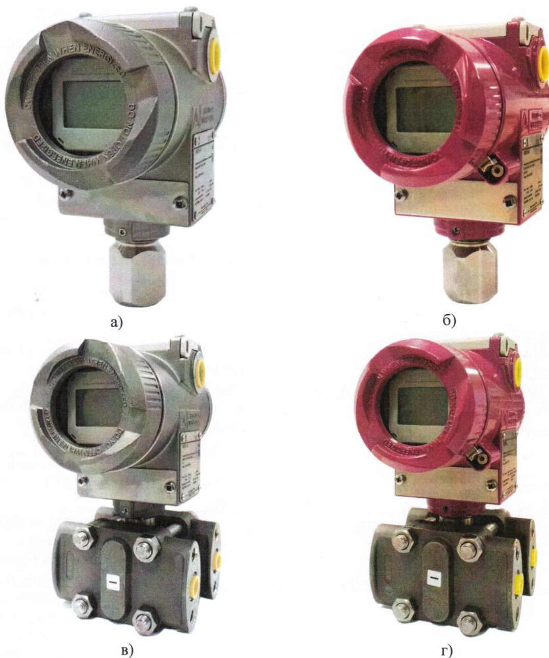
Рисунок 1 - Общий вид преобразователей (а, в - KM35 в нержавеющей корпусе; б, г - KM35 в корпусе из алюминия)
